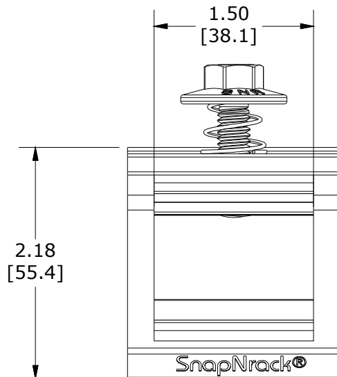
TOP
