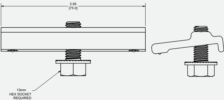
MLPE Mount, Module
