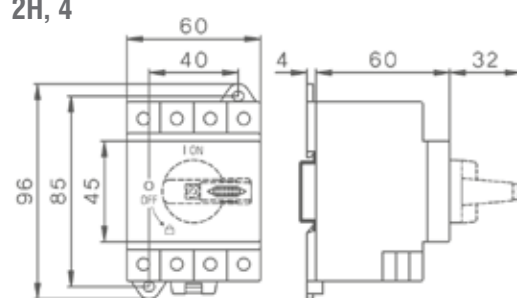
SI40DB(L) / SI55DB(L)
