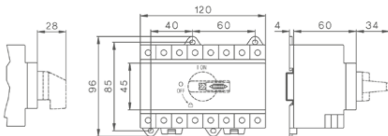
SI16DB(L) / SI25DB(L) / SI32DB(L) / SI38DB(L)
