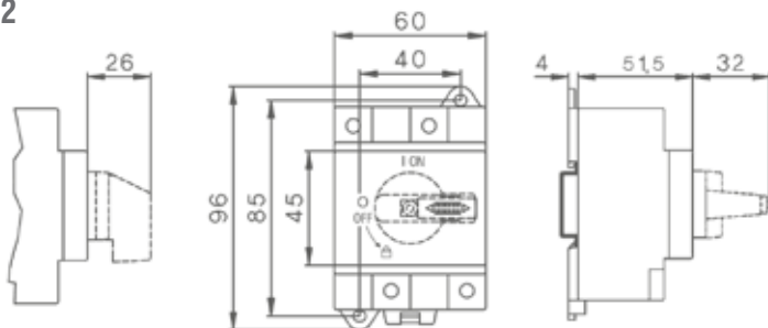
SI40DB(L) / SI55DB(L)
