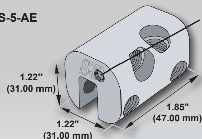
SnoPost E
