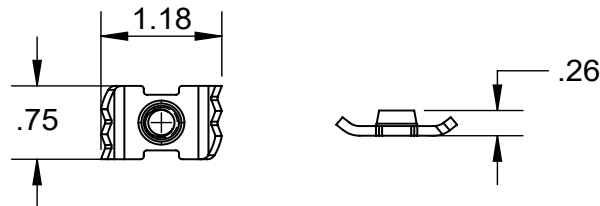
3) T-Nut, Sheet Metal
